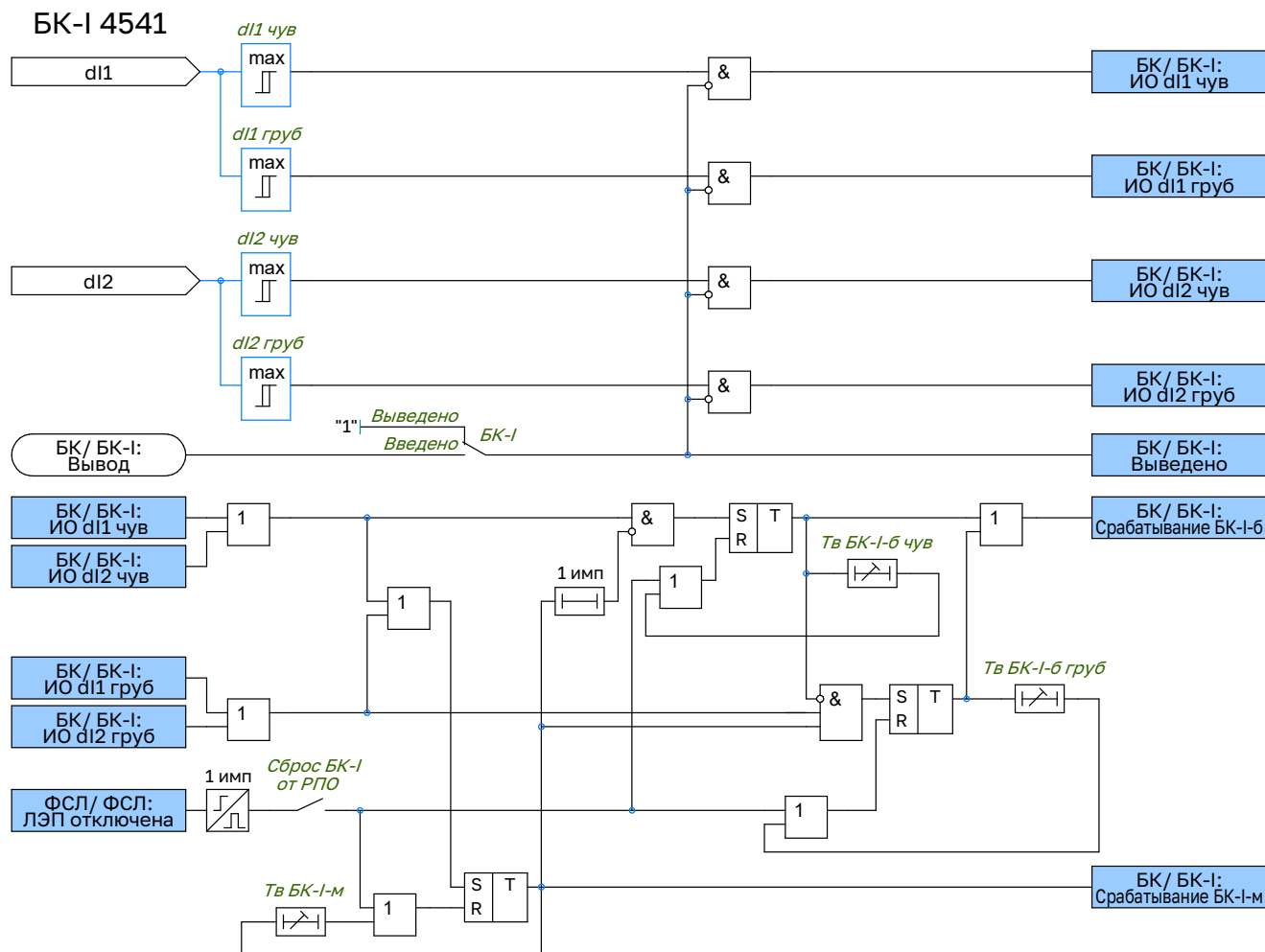
Рисунок 1.15 – Функциональная схема пуска БК-I
