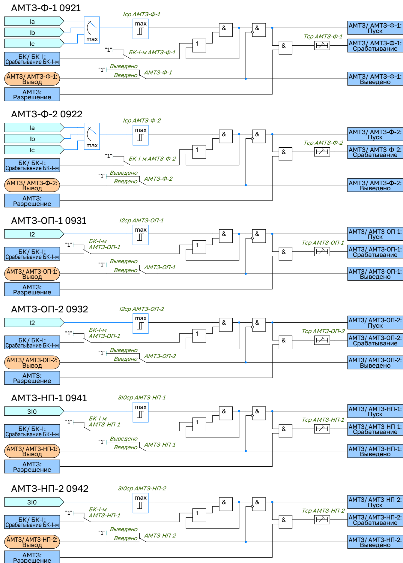
Рисунок 1.25 – Функциональная схема ступеней AMT3-Φ-1(2)
