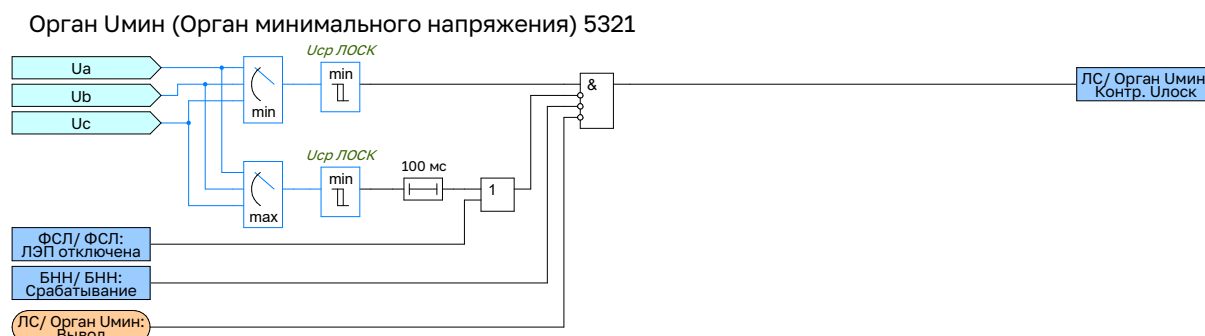
Рисунок 1.36 – Функциональная схема логики контроля минимального напряжения ЛОСК
