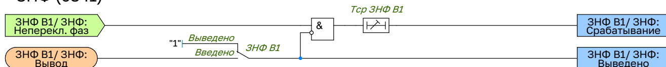
Рисунок 1.28 – Функциональная схема ЗНФ В1
