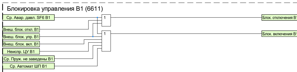
Рисунок 1.47 – Функциональная схема блокировки управления В1
