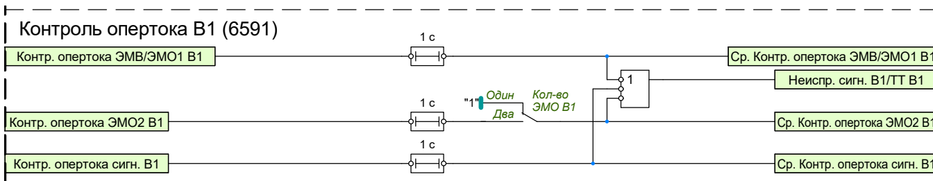
Рисунок 1.45 – Функциональная схема контроля опертока В1
