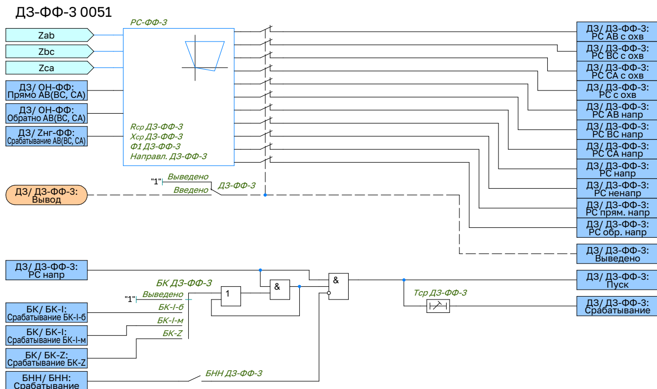
Рисунок 1.9 – Функциональная схема логики ДЗ-ФФ-3
