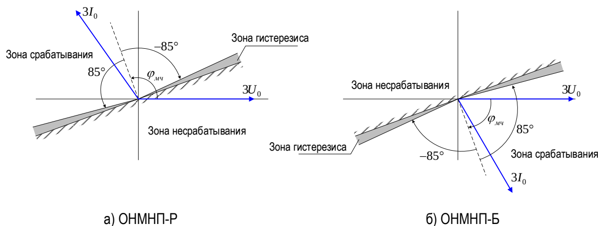
Рисунок 1.19 – Характеристики срабатывания ОНМНП
