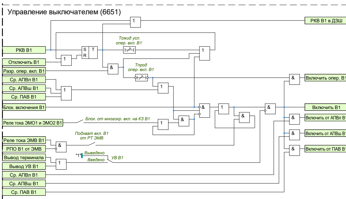
Рисунок 1.51 – Функциональная схема управления выключателем В1
