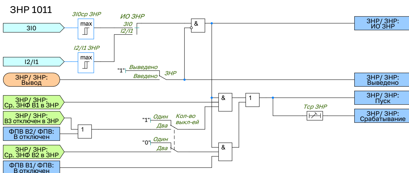
Рисунок 1.29 – Функциональная схема ЗНР
