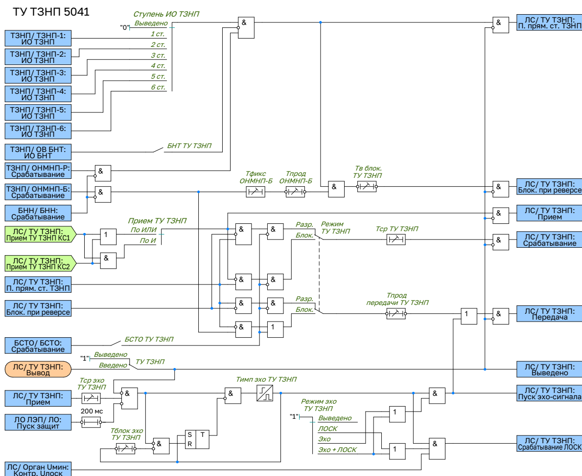
Рисунок 1.37 – Функциональная схема ТУ ТНЗНП
