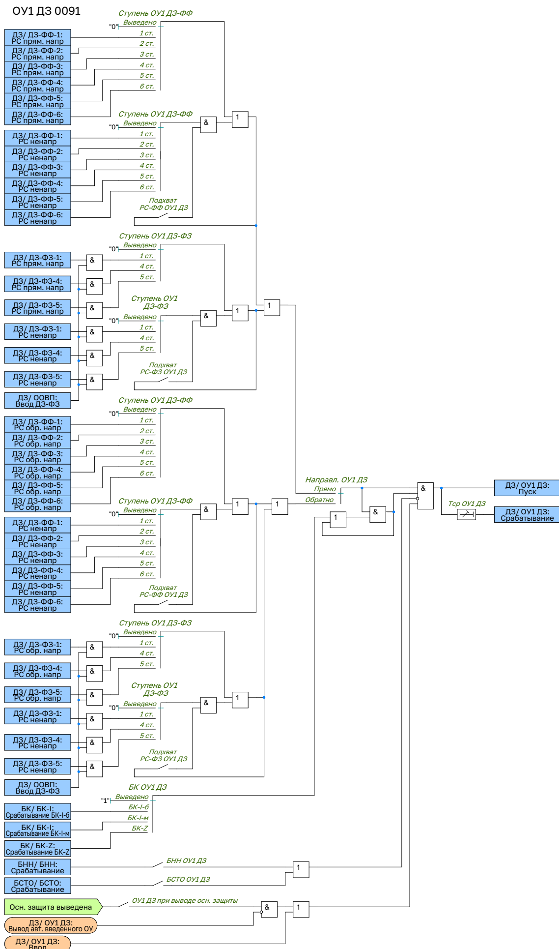
Рисунок 1.13 – Функциональная схема логики ОУ ДЗ
