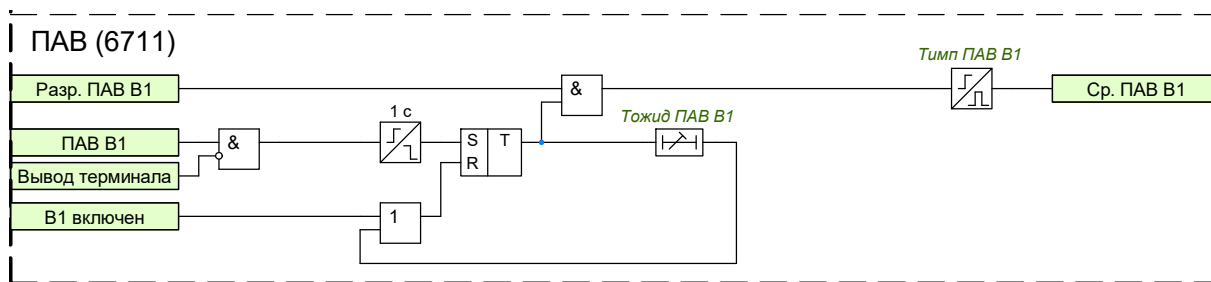
Рисунок 1.42 – Функциональная схема логики ПАВ В1
