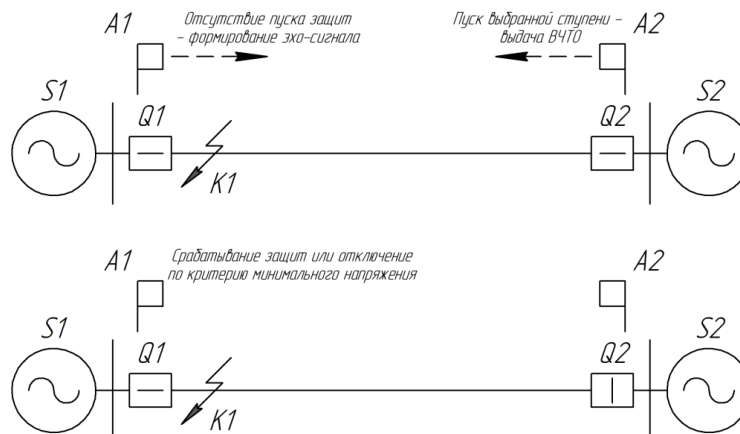
Рисунок 1.35 – Пояснение к принципу действия эхо-логики
