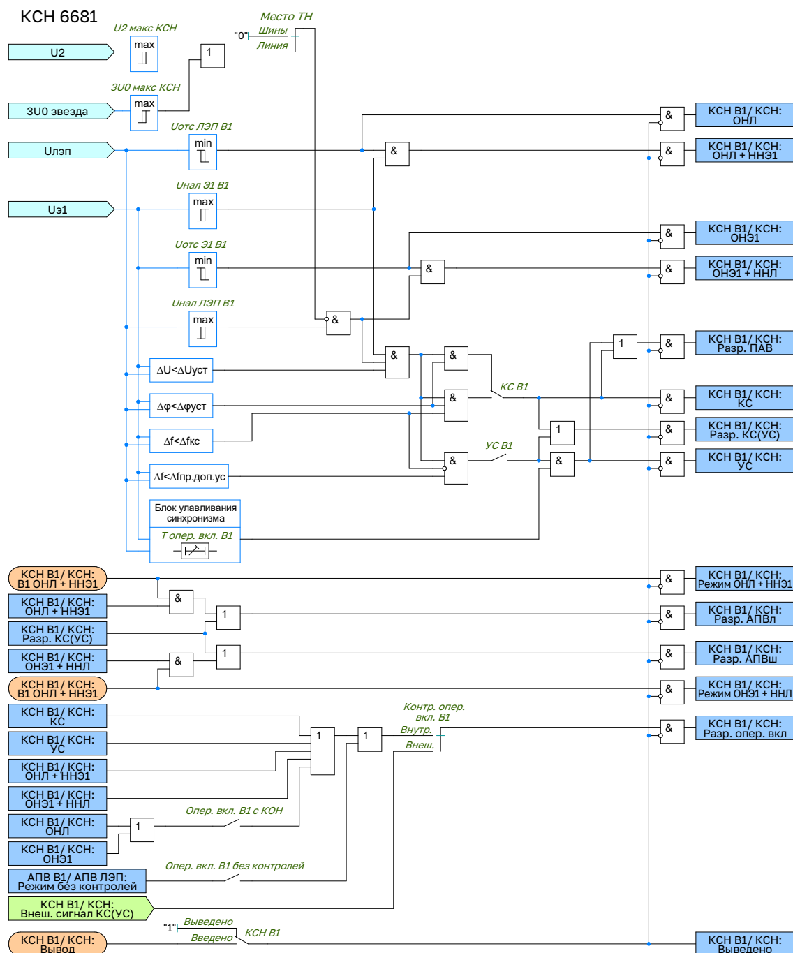
Рисунок 1.39 – Функциональная схема логики КСН В1
