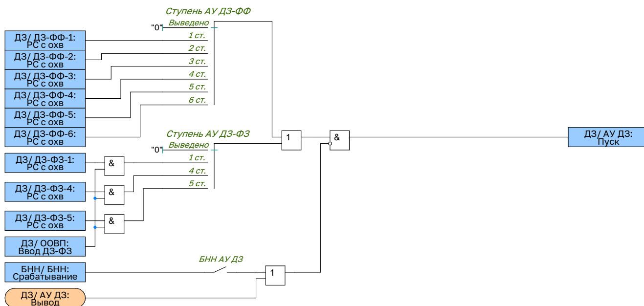
Рисунок 1.12 – Функциональная схема пуска АУ ДЗ
