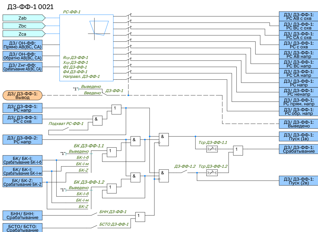
Рисунок 1.7 – Функциональная схема логики ДЗ-ФФ-1
