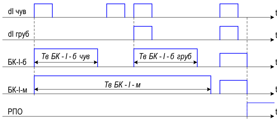
Рисунок 1.14 – Временная диаграмма работы БК-I
