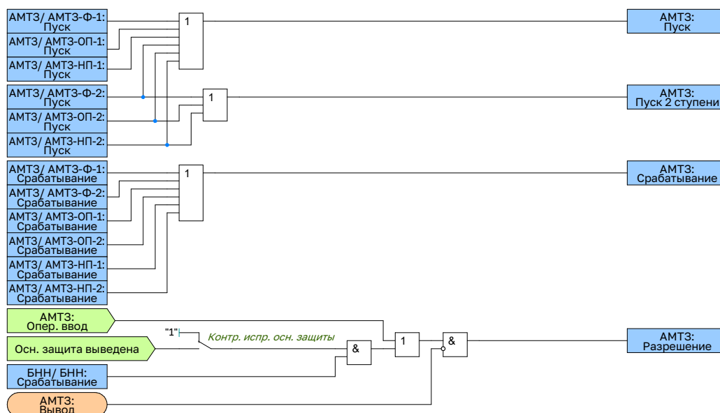
Рисунок 1.24 – Функциональная схема общей логики АМТЗ
