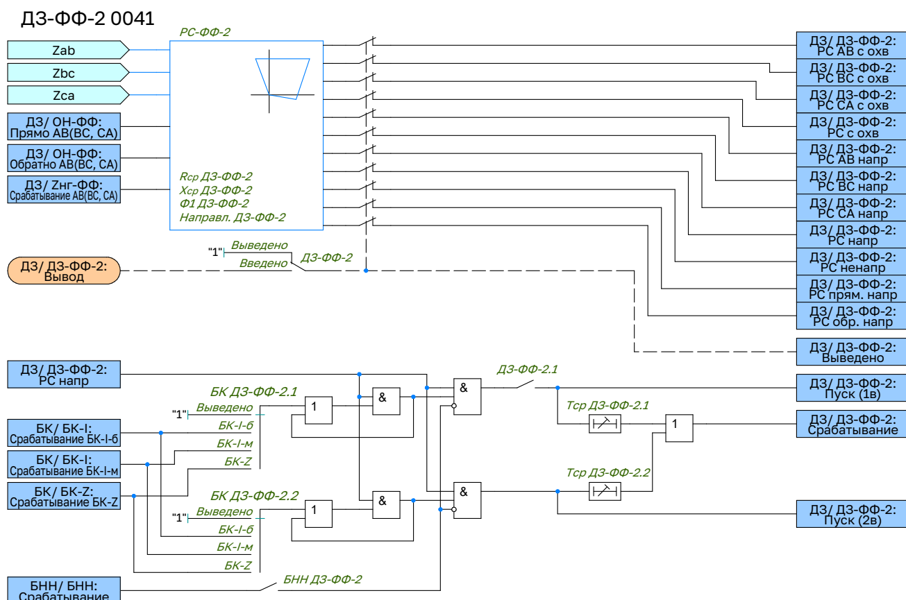
Рисунок 1.8 – Функциональная схема логики ДЗ-ФФ-2
