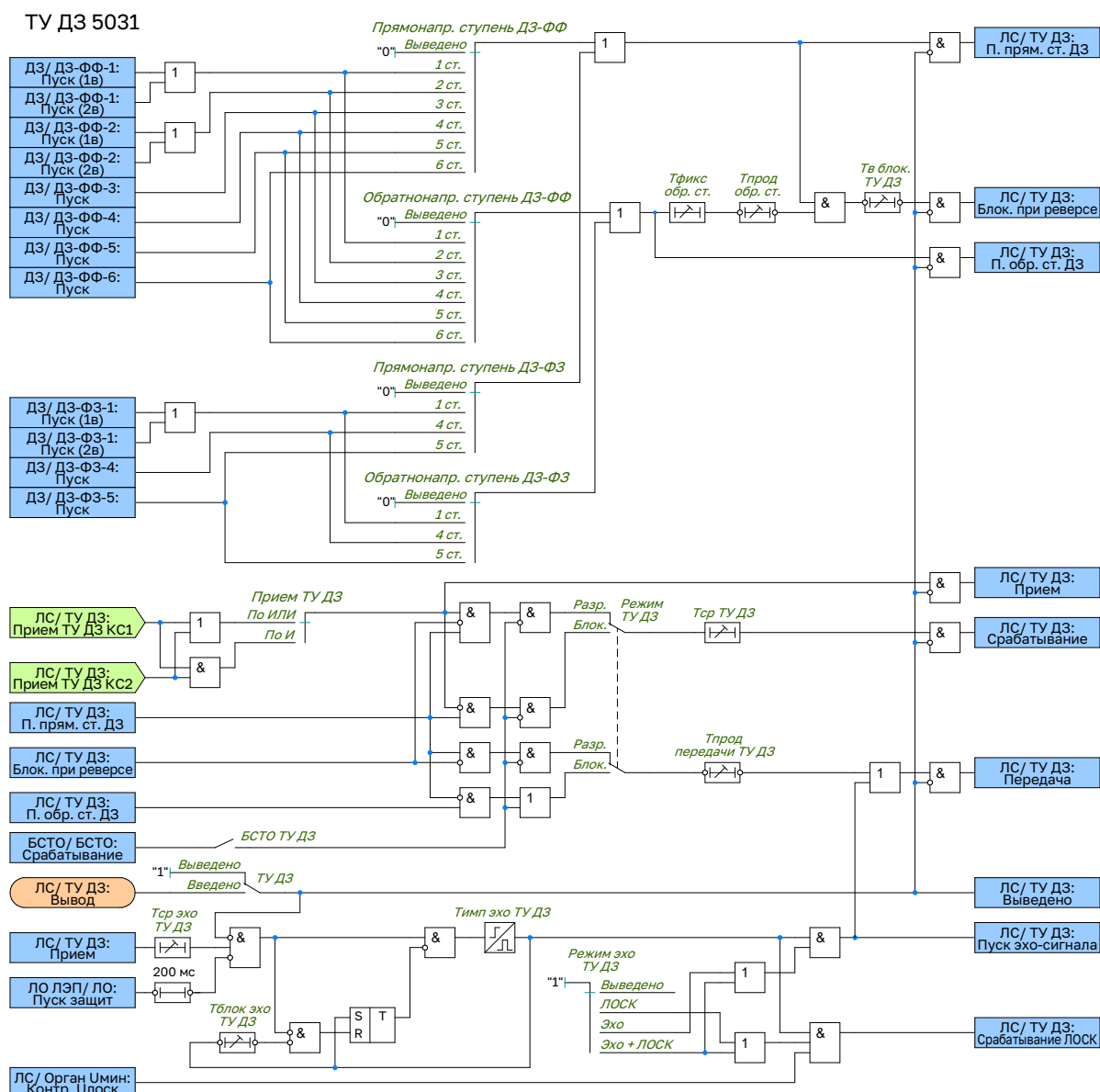
Рисунок 1.34 – Функциональная схема логики ТУ ДЗ
