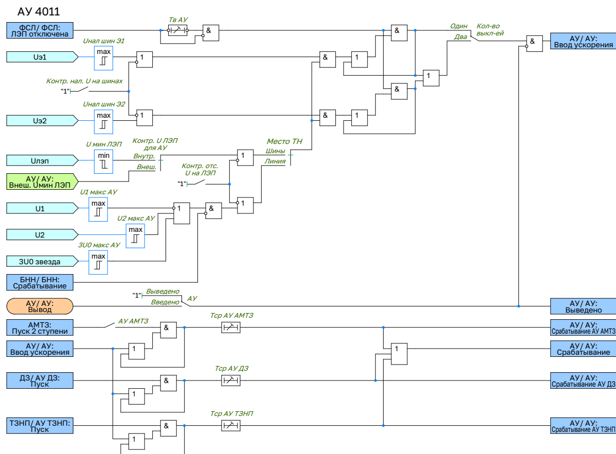
Рисунок 1.31 – Функциональная схема АУ
