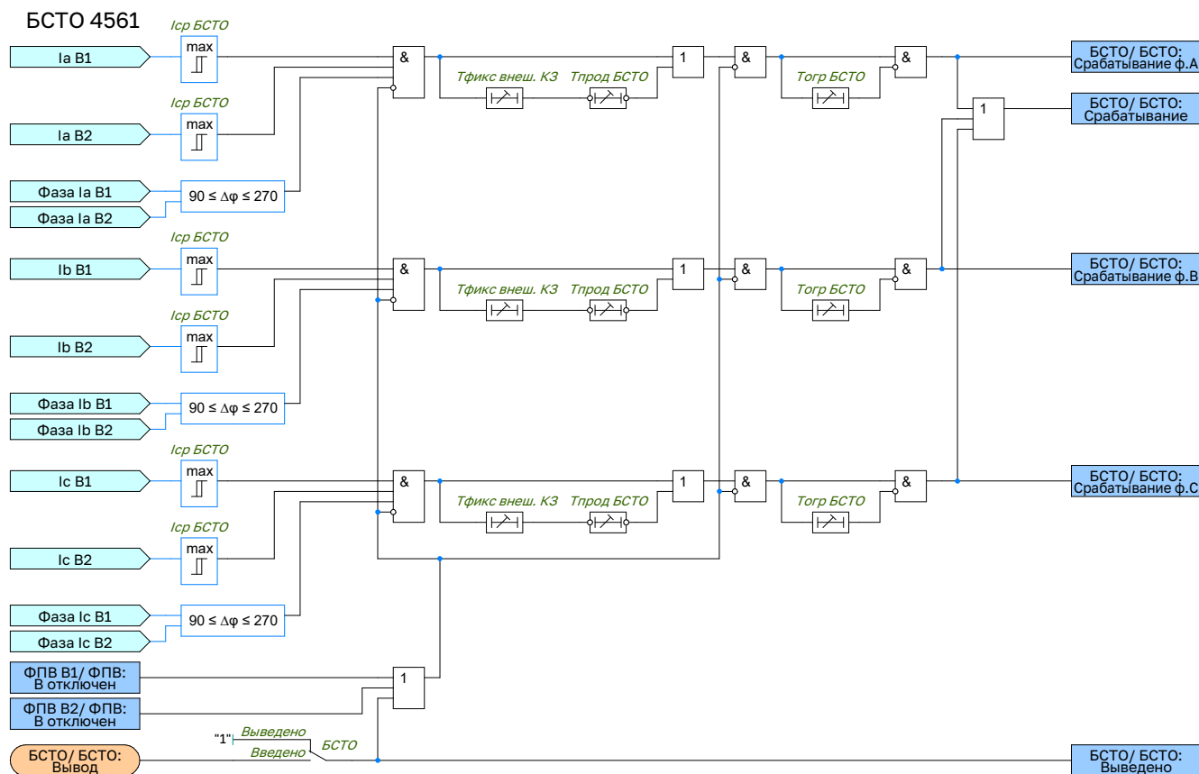
Рисунок 1.27 – Функциональная схема БСТО
