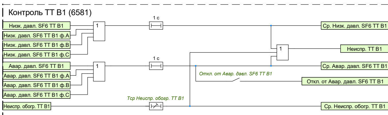
Рисунок 1.44 – Функциональная схема контроля ТТ В1
