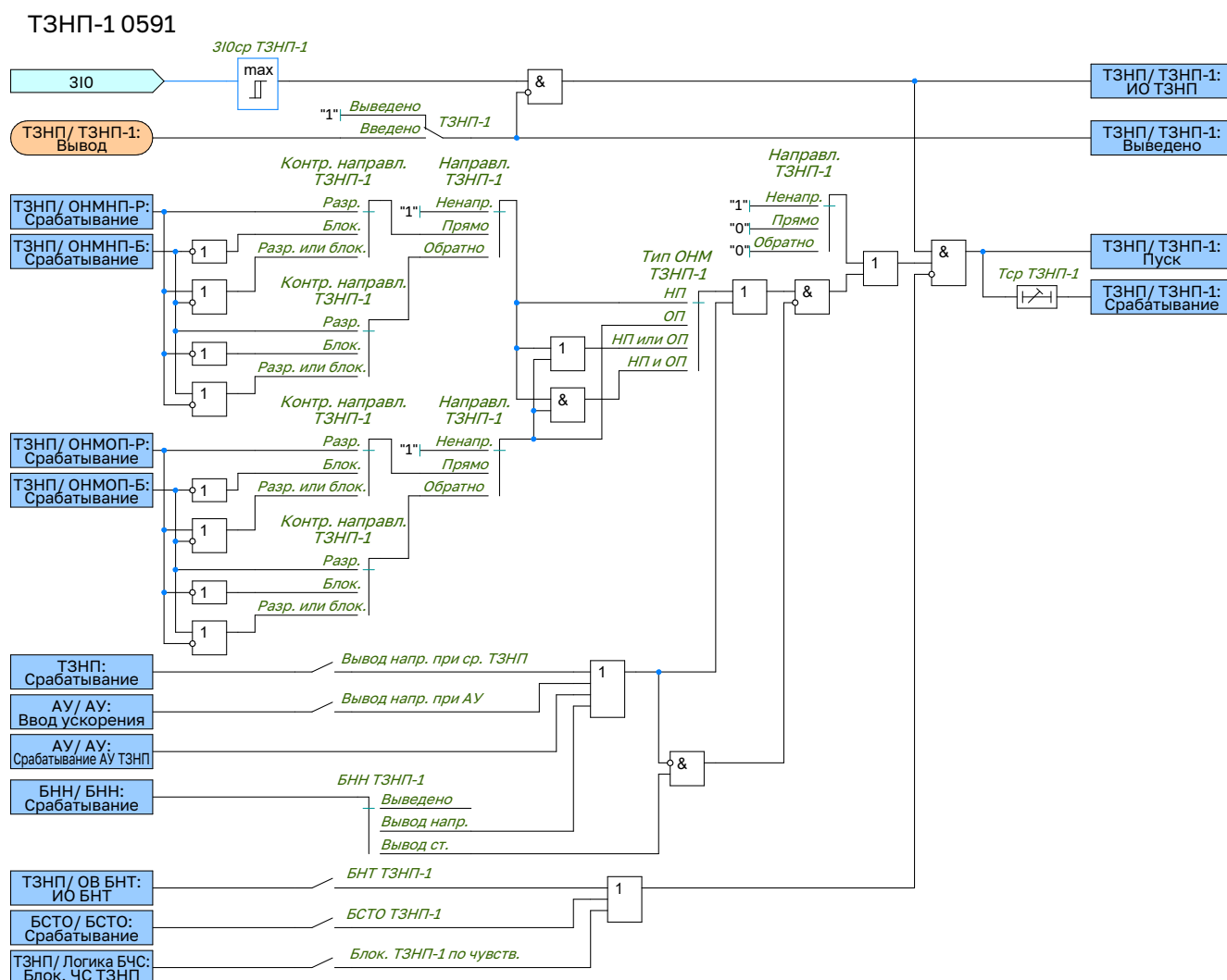
Рисунок 1.18 – Функциональная схема ступени ТНЗНП-1
