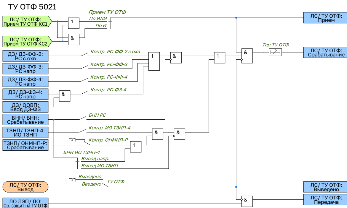
Рисунок 1.33 – Функциональная схема логики ТУ ОТФ
