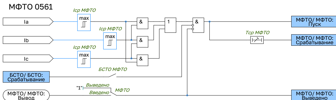
Рисунок 1.23 – Функциональная схема МФТО
